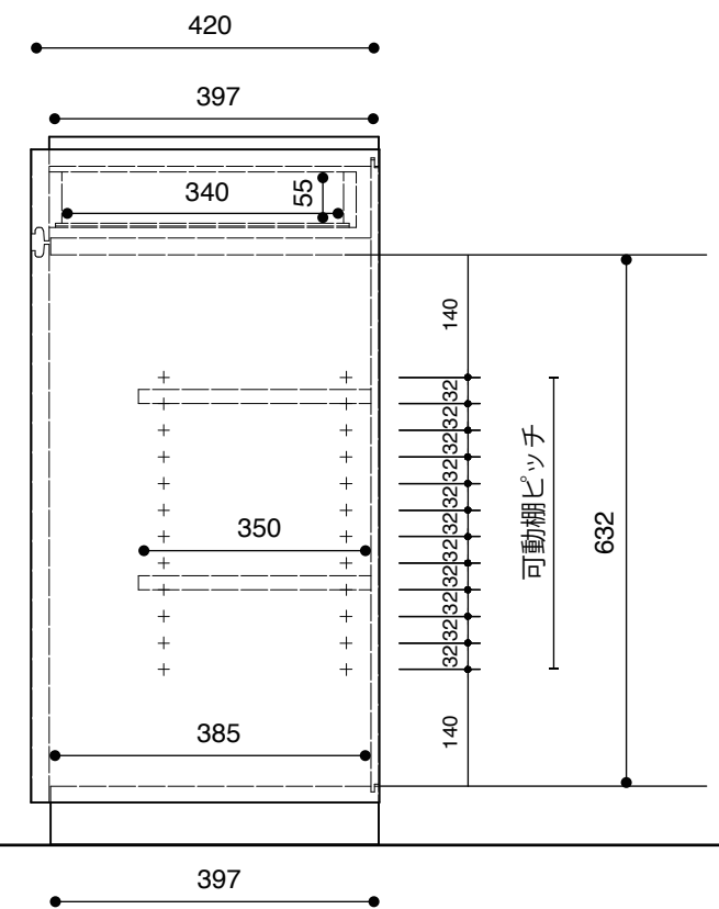
【側面】
