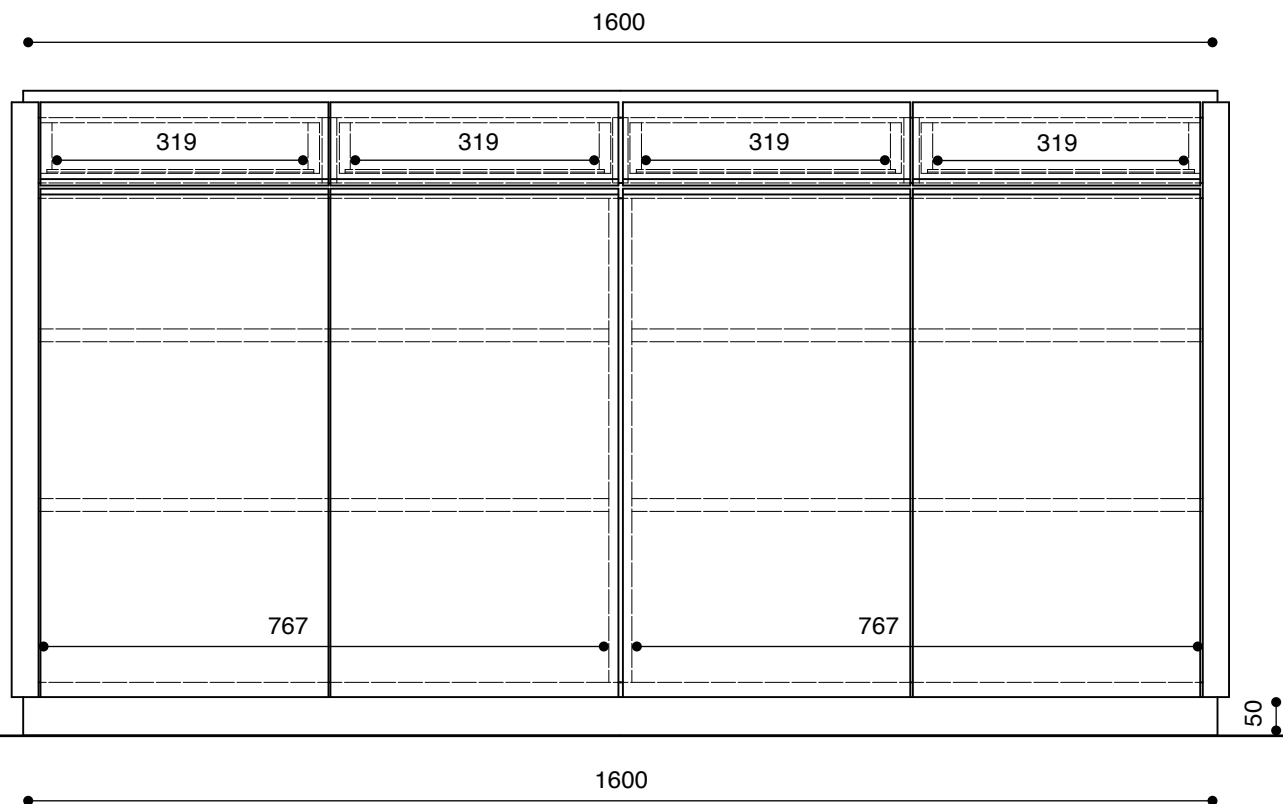
【正面】
